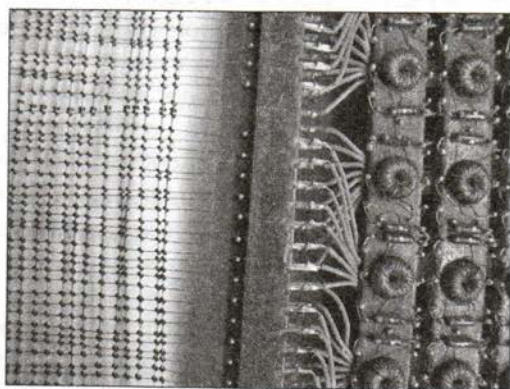
Рис. 5.13. Магнитное ОЗУ:
