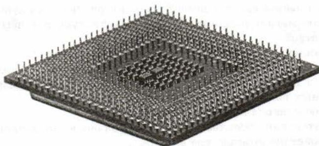
Рис. 5.11. Вид микропроцессора со стороны выводов
