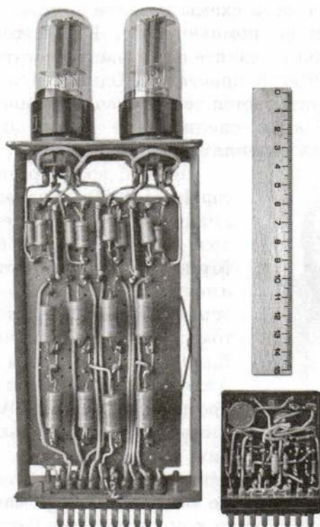
Рис. 5.5. Уменьшение размеров ячеек памяти ЭВМ от первого до третьего поколений (в каждой из них — по два триггера)
